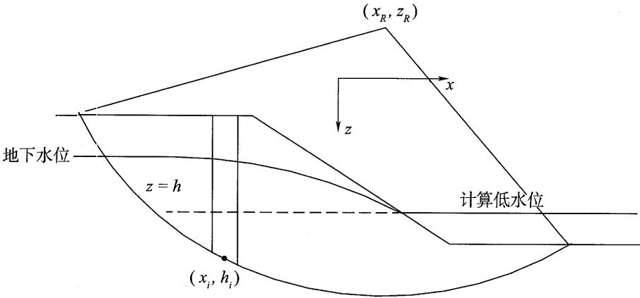
图 4.6.4 稳定验算示意图
