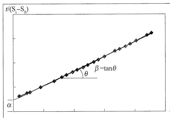
图 B.0.1 \alpha, \beta 值确定示意图
