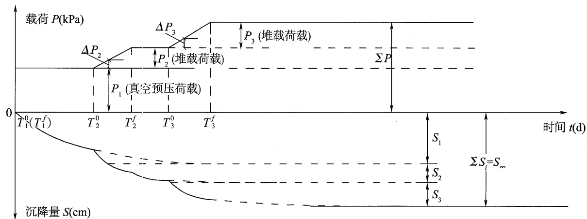
图 4.6.1 分级加荷固结过程示意图
