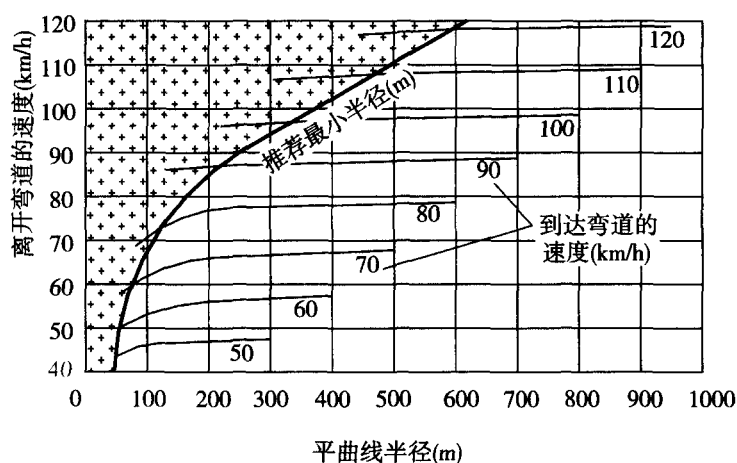
图 B(2)0.1-2 曲线段小客车的运行速度
