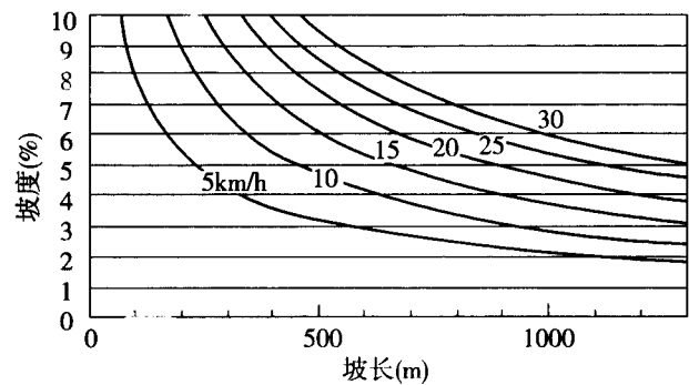
图 B(1).0.2 速度折减量与坡长的关系曲线图
