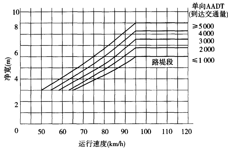
图 C.0.1-1 填方路基安全净宽
