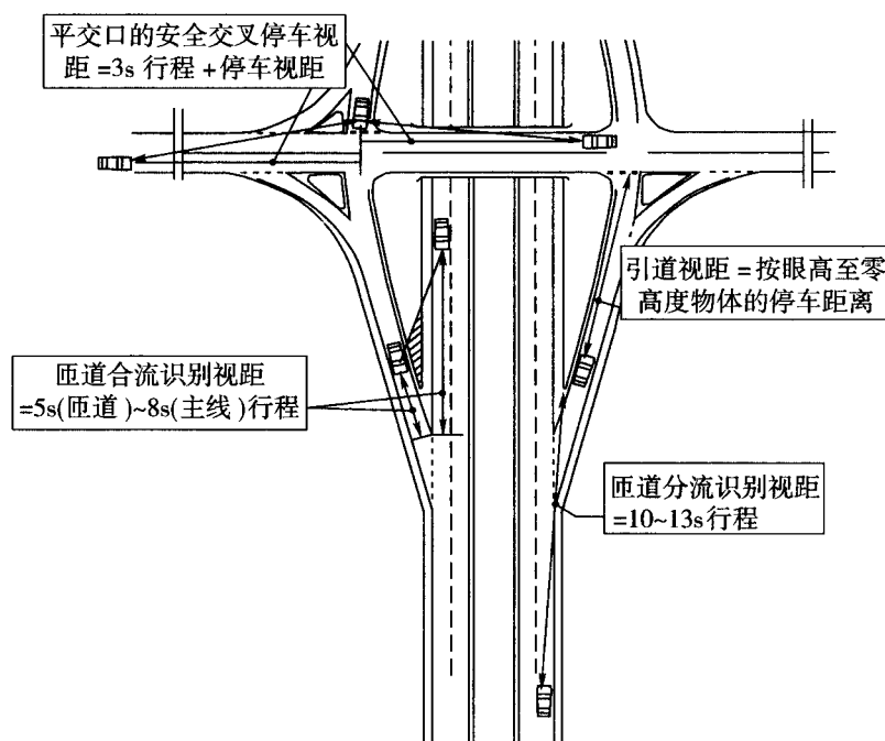
图 4.6.2 互通式立交视距参数图
