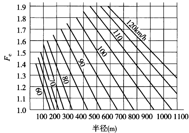
图 C.0.2 曲线段安全净空带宽度调整系数
