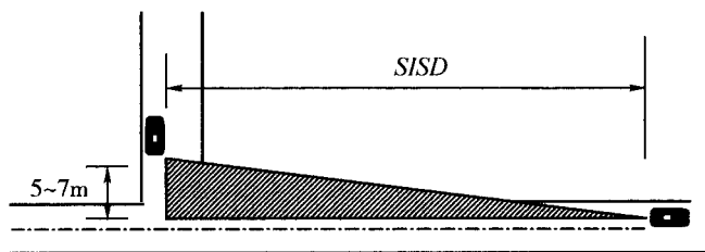
图 4.6.1-2 安全交叉停车视距三角区
