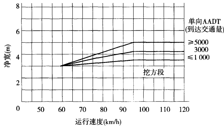
图 C.0.1-2 挖方路基安全净宽
